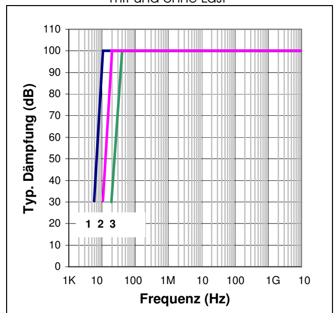
Einfügungs-Dämpfung nach CISPR 17
