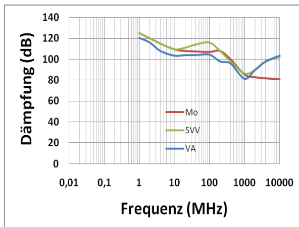
Schirmdämpfung im H-Feld
