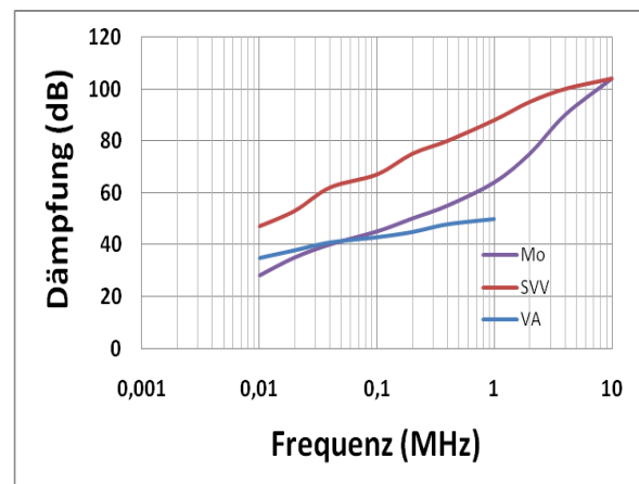
Schirmdämpfung im E-Feld
