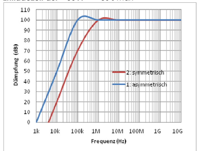
Einfügungs-Dämpfung nach CISPR 17 in 50 Ω-Systemen, mit und ohne Last
