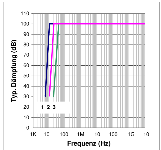
Einfügungs-Dämpfung nach CISPR 17 in 50 \Omega -Systemen, asymmetrisch, mit und ohne Last
